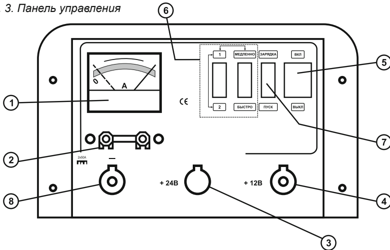
Рис. 3. Панель управления
