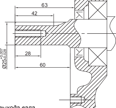
Рис. 1. Двигатель в сборе и схема выхода вала
