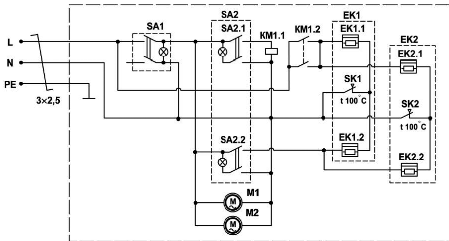
EK1, EK 2 - электронагреватели; KM1 - магнитный пускатель; M1, M2 - электродвигатели вентилятора; SA1 - сетевой переключатель; SA2 - переключатель режимов нагрева; SK1, SK2 - термopедохранители;
