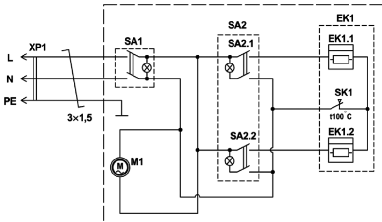
EK1 - электронагреватель; M1 - электродвигатель; SA1 - сетевой переключатель; SA2 - переключатель режимов нагрева; SK1 - термopедохранитель; XP1 - вилка сетевая;
